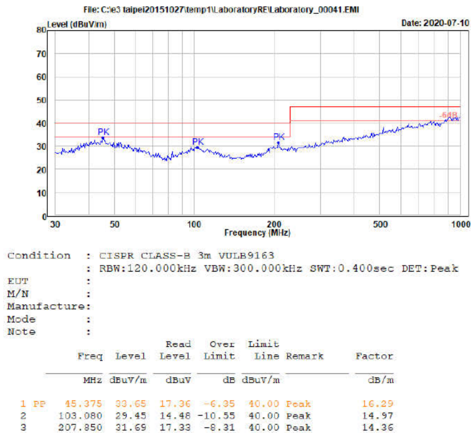
图 3-7 辐射测试垂直方向
