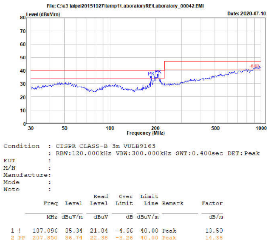
图 3-6 辐射测试水平方向
