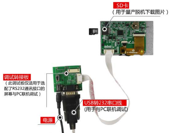
图 1-5 调试工具图
