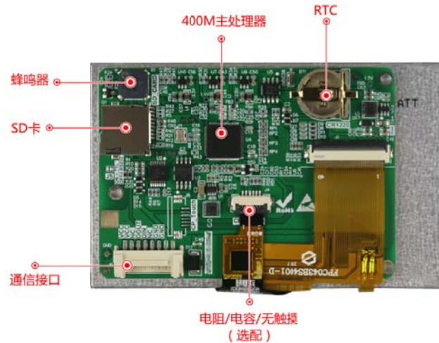
图 1-4 硬件配置图
