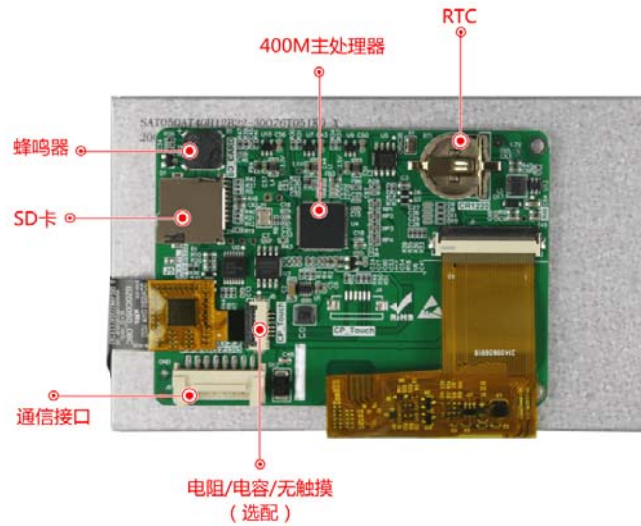
图 1-4 硬件配置图
