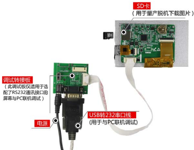
图 1-5 调试工具图
