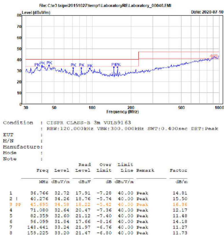
图 3-7 辐射测试垂直方向
