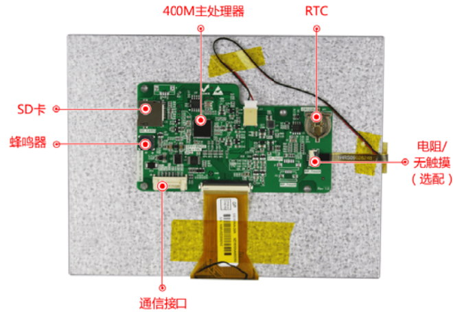
图 1-3 硬件配置图
