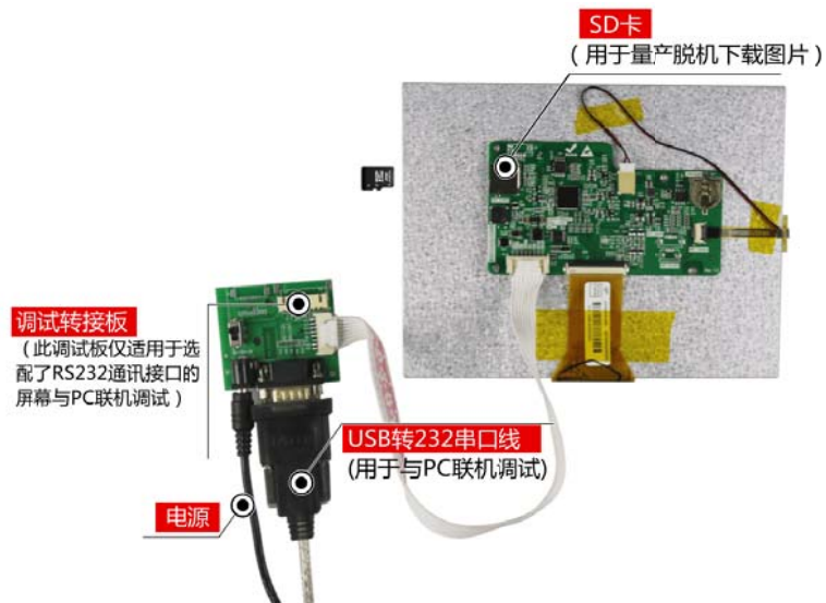
图 1-4 调试工具图
