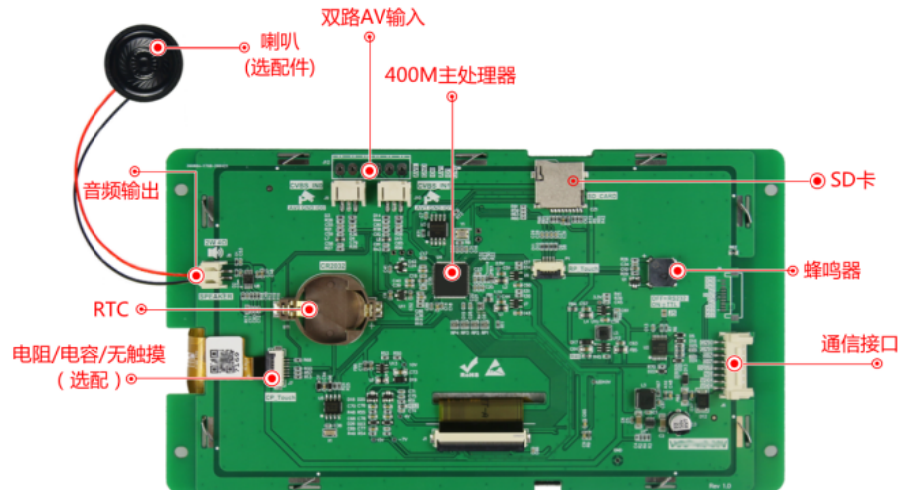
图 1-4 硬件配置图
