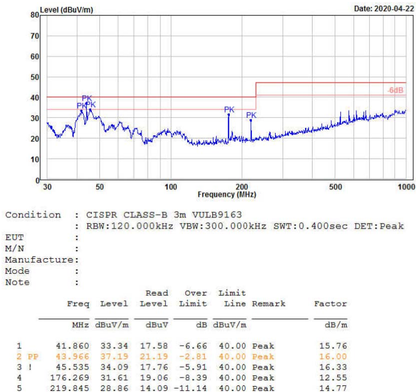
图 3-7 辐射测试垂直方向
