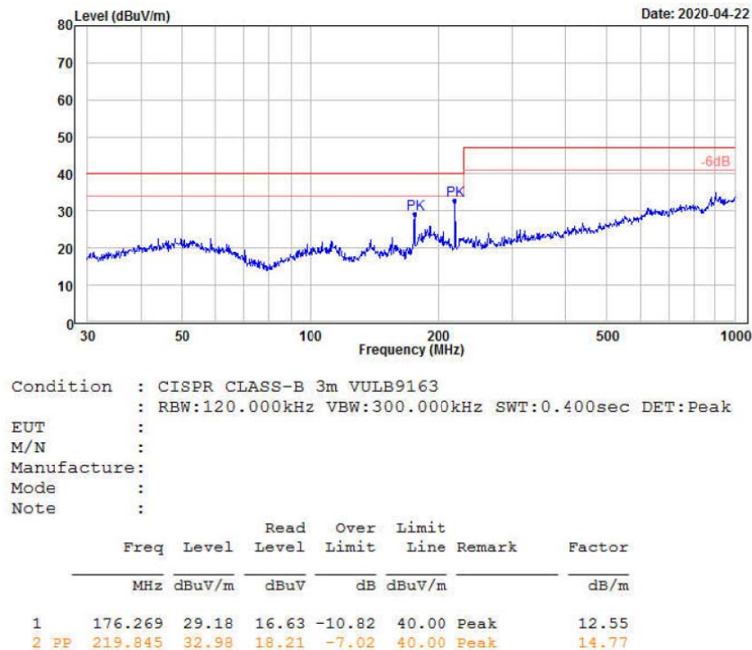
图 3-6 辐射测试水平方向
