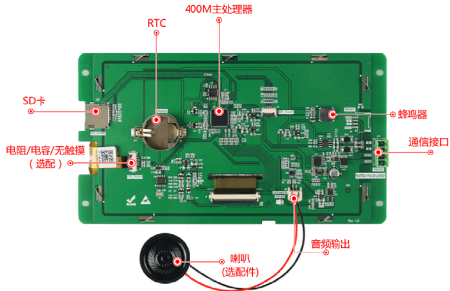
图 1-4 硬件配置图
