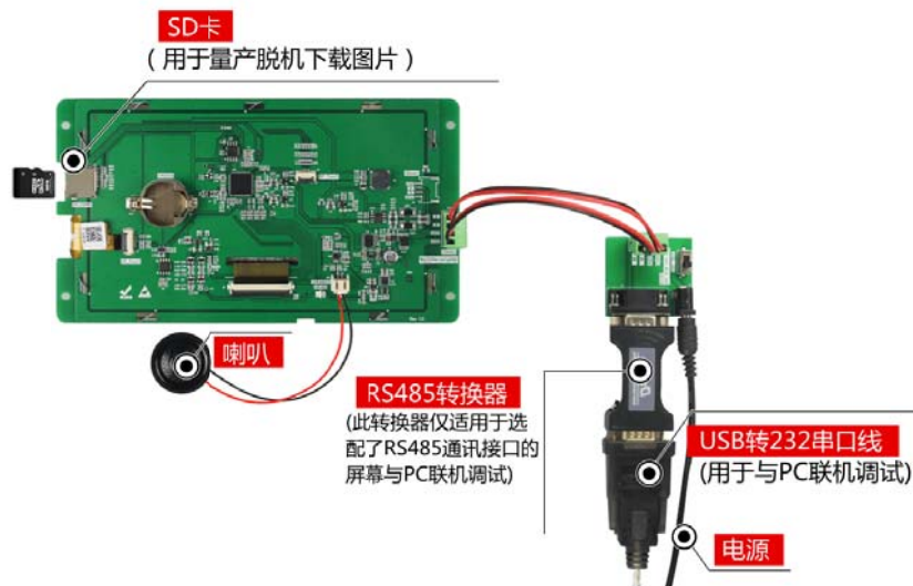
图 1-5 调试工具图
