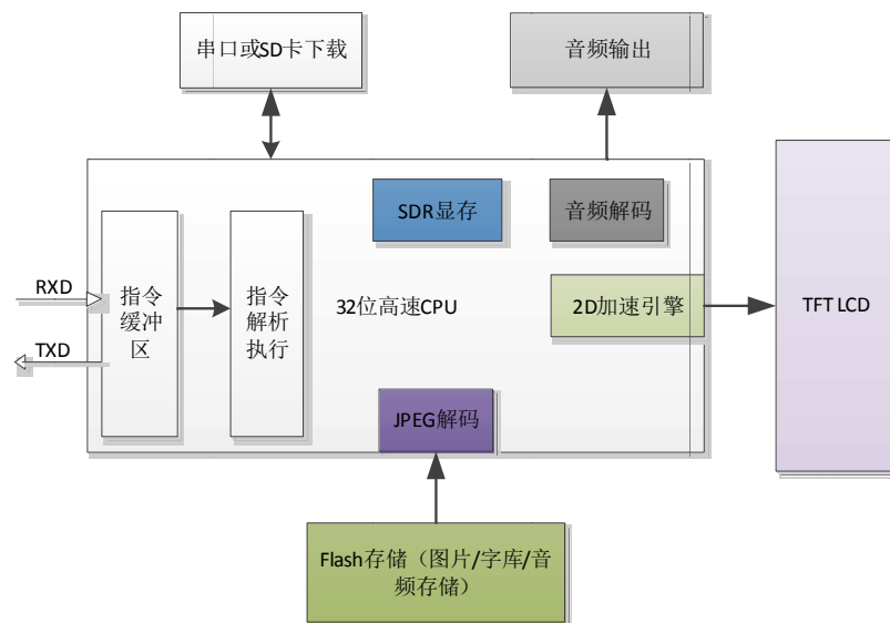
图 9-1 M 系列串口屏内部结构图
