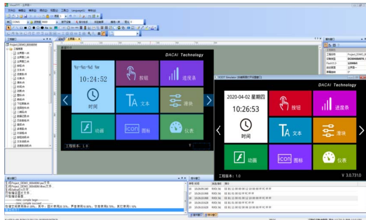
图 10-1 VisualTFT 主界面
