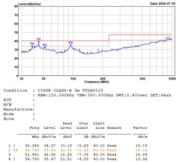
图 3-7 辐射测试垂直方向
