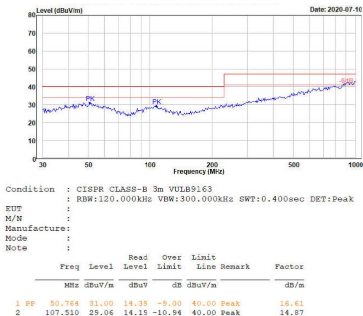
图 3-6 辐射测试水平方向
