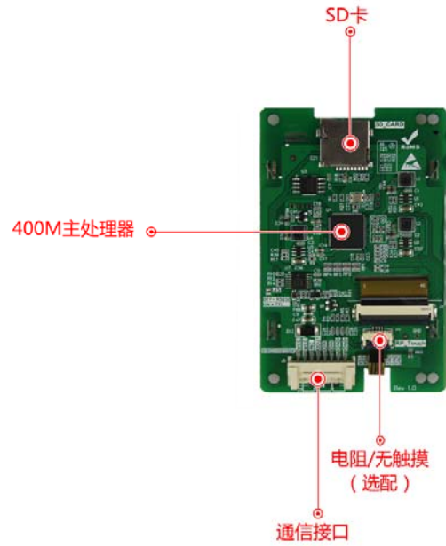
图 1-3 硬件配置图
