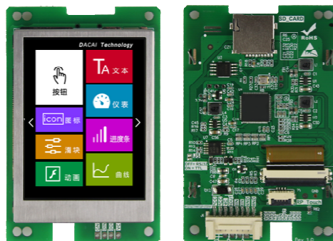
图 1-2 2.8 寸无触摸参考图
