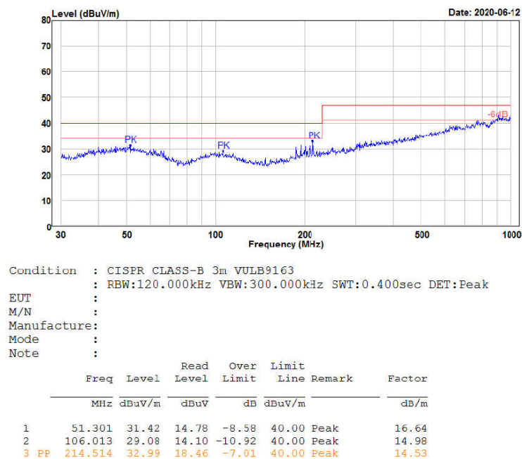
图 3-6 辐射测试水平方向
