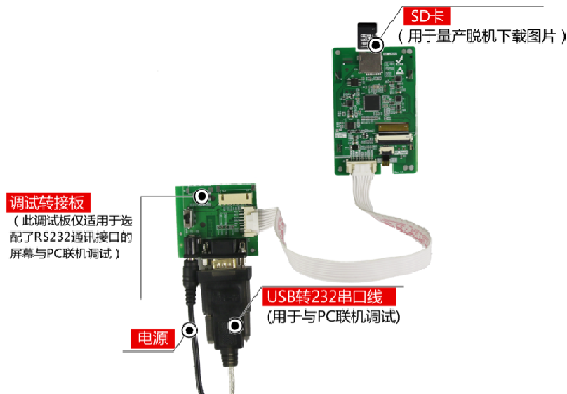
图 1-4 调试工具图
