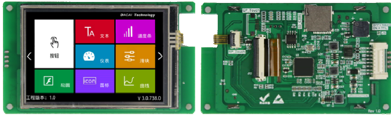
图 1-1 3.5 寸电阻触摸参考图
