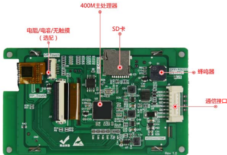
图 1-4 硬件配置图
