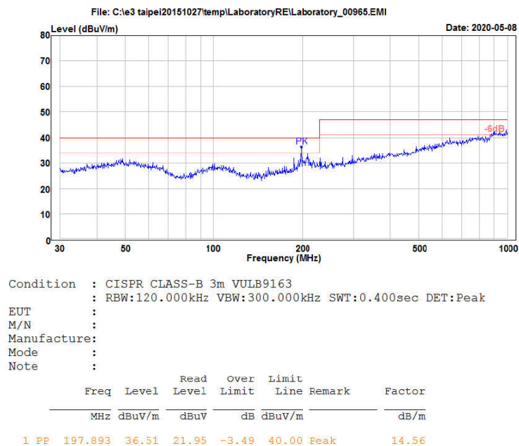
图 3-6 辐射测试水平方向
