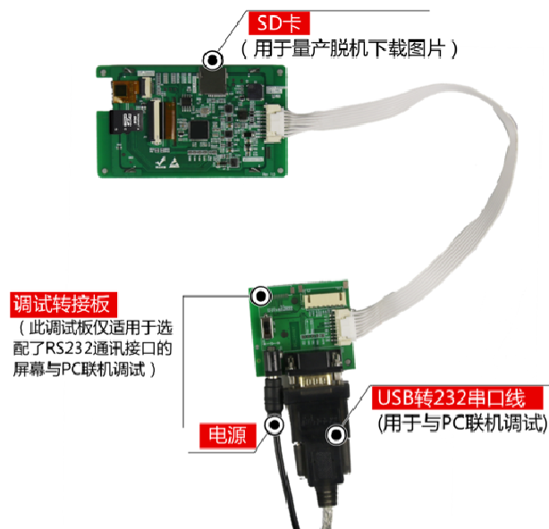
图 1-5 调试工具图
