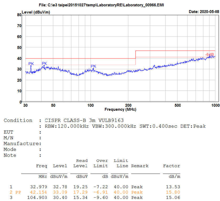
图 3-7 辐射测试垂直方向
