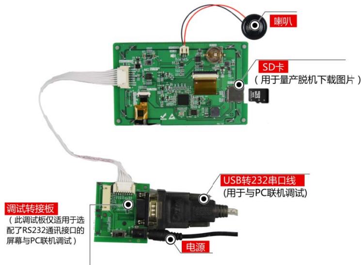
图 1-5 调试工具图
