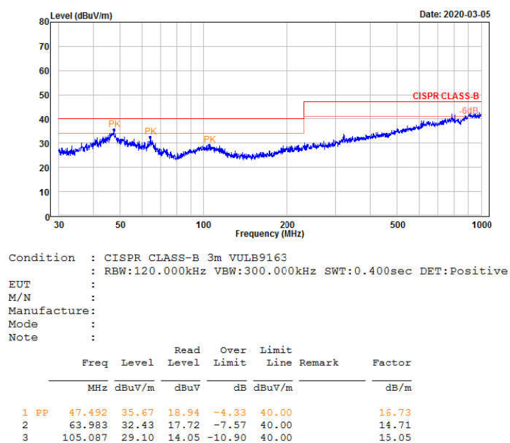
图 3-7 辐射测试垂直方向
