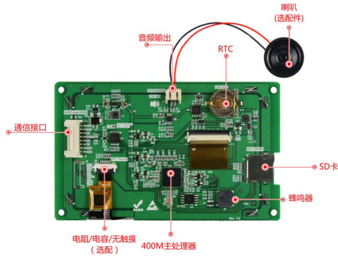
图 1-4 硬件配置图
