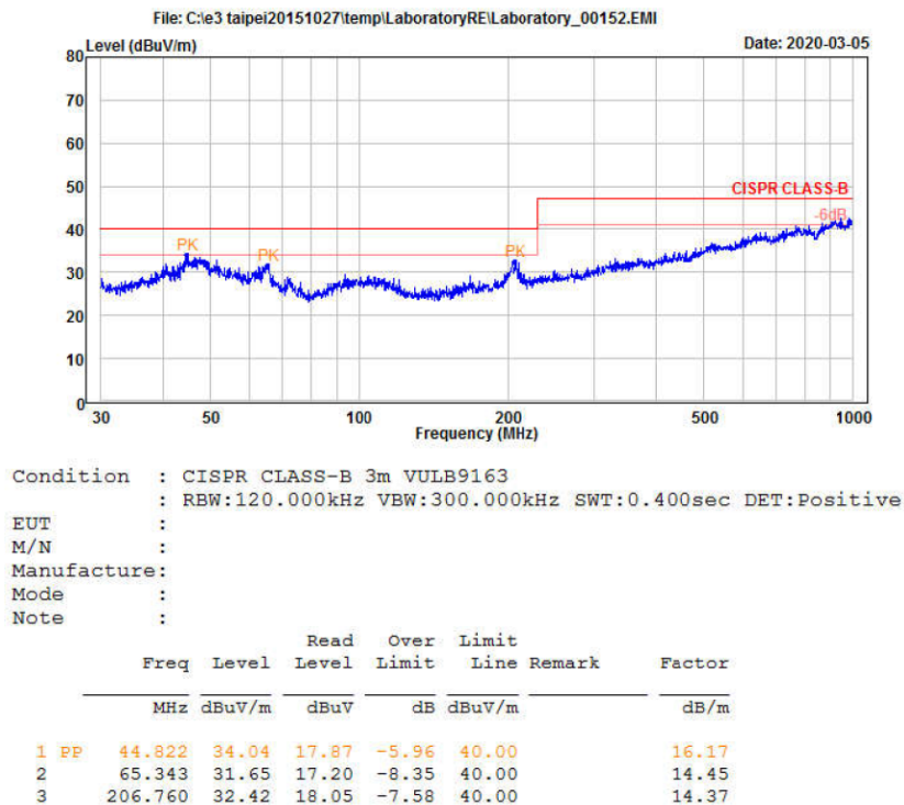
图 3-7 辐射测试垂直方向
