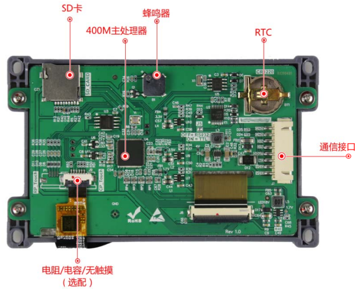
图 1-4 硬件配置图
