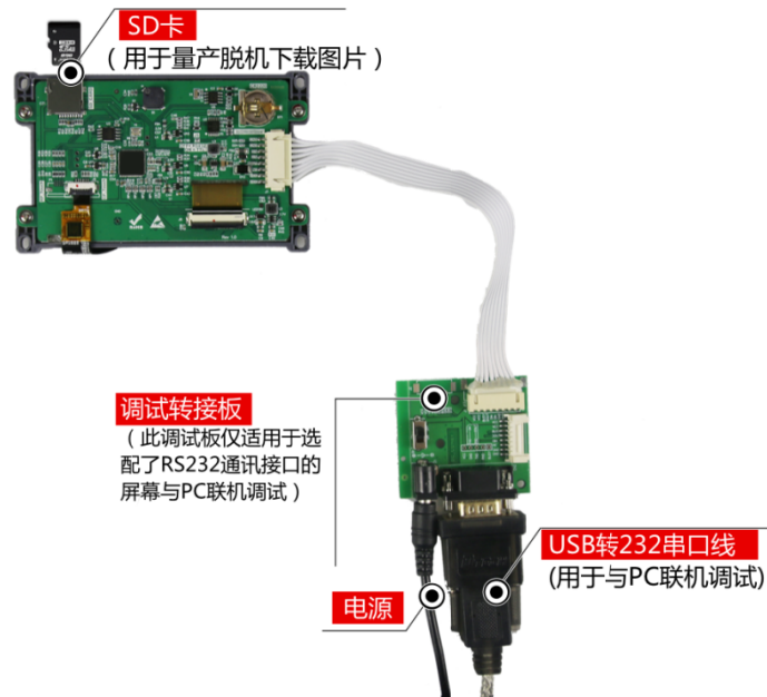
图 1-5 调试工具图
