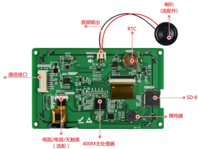
图 1-4 硬件配置图
