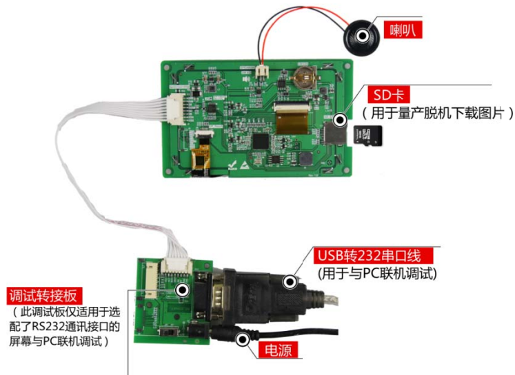
图 1-5 调试工具图
