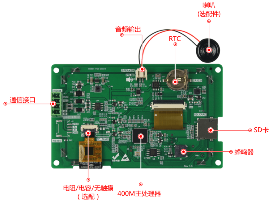
图 1-4 硬件配置图
