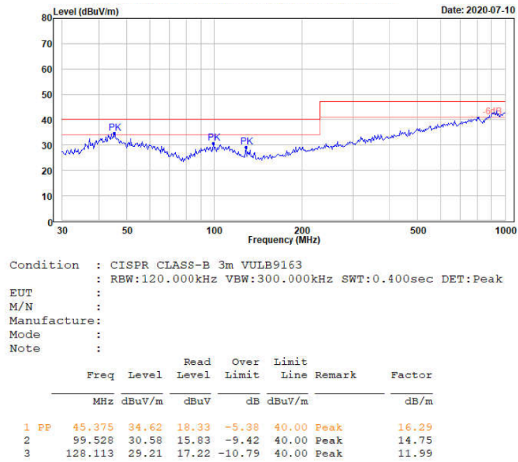
图 3-7 辐射测试垂直方向
