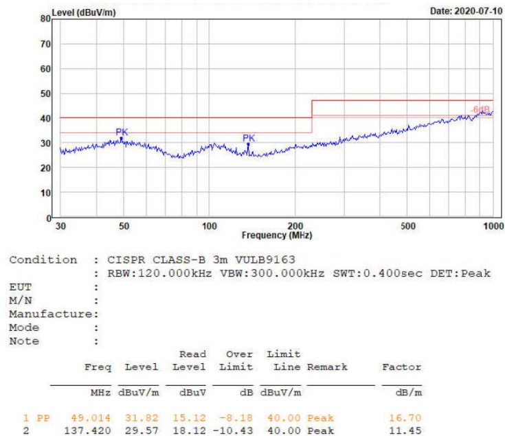
图 3-6 辐射测试水平方向
