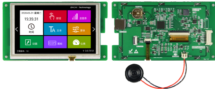
图 1-1 5.0 寸电阻触摸参考图
