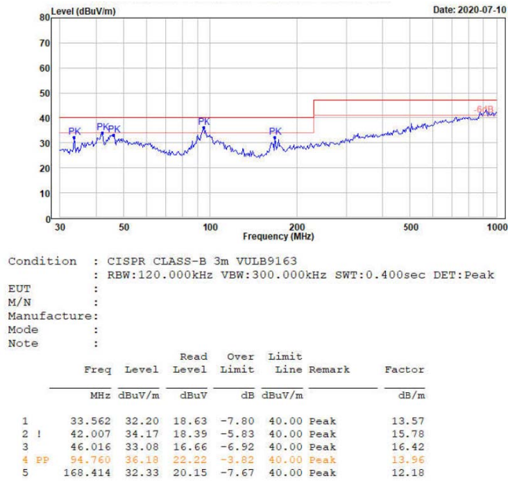
图 3-7 辐射测试垂直方向
