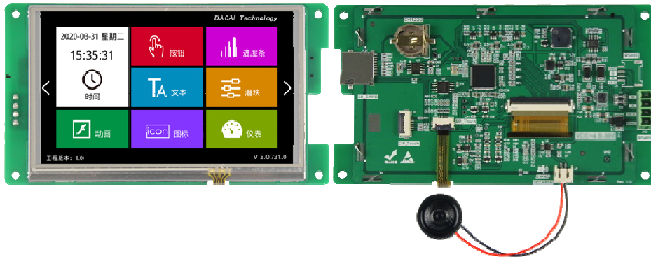
图 1-1 5.0 寸电阻触摸参考图
