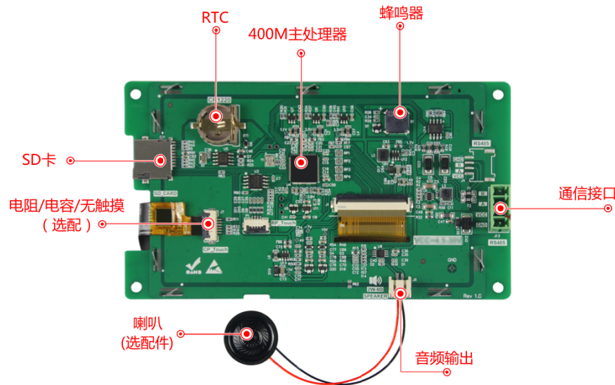
图 1-4 硬件配置图
