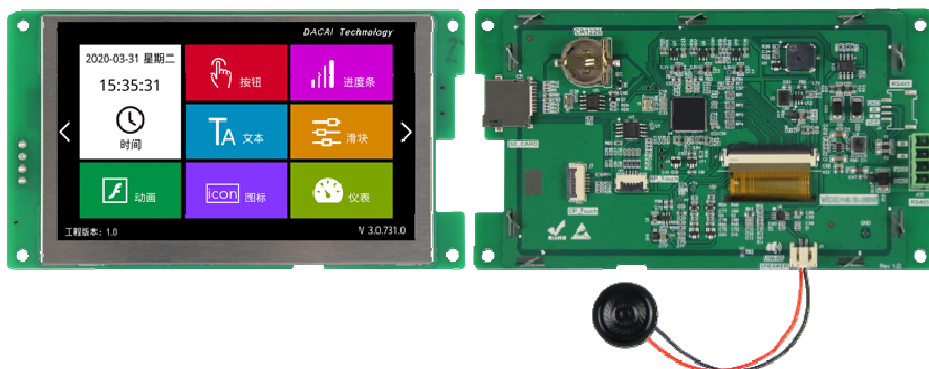
图 1-3 5.0 寸无触摸参考图
