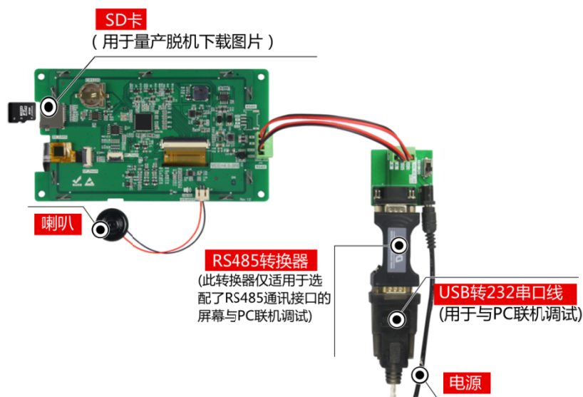
图 1-5 调试工具图
