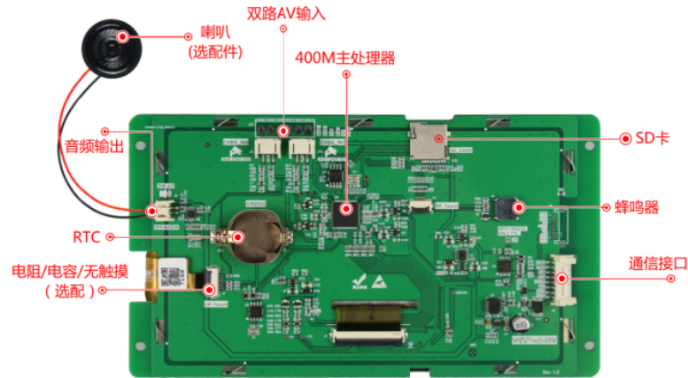
图 1-4 硬件配置图
