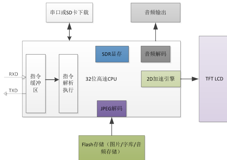
图 10-1 GM 系列串口屏内部结构图
