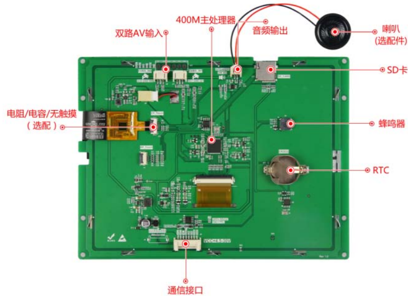
图 1-4 硬件配置图
