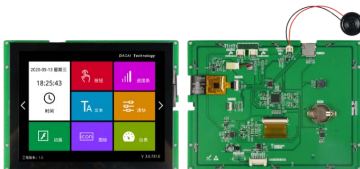
图 1-2 8.0 寸电容触摸参考图
