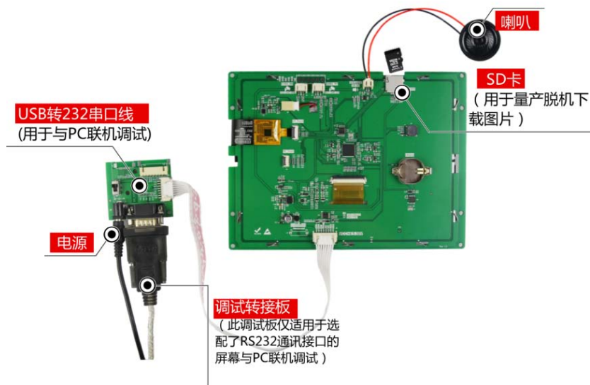
图 1-5 调试工具图
