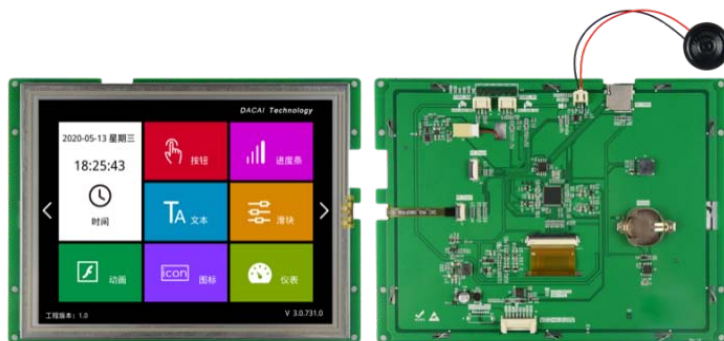
图 1-1 8.0 寸电阻触摸参考图
