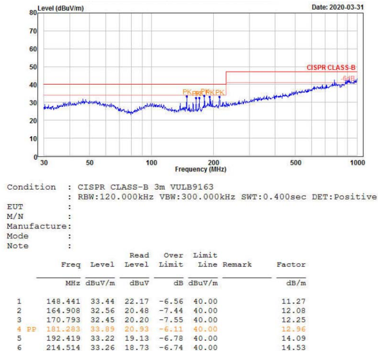
图 3-6 辐射测试水平方向
