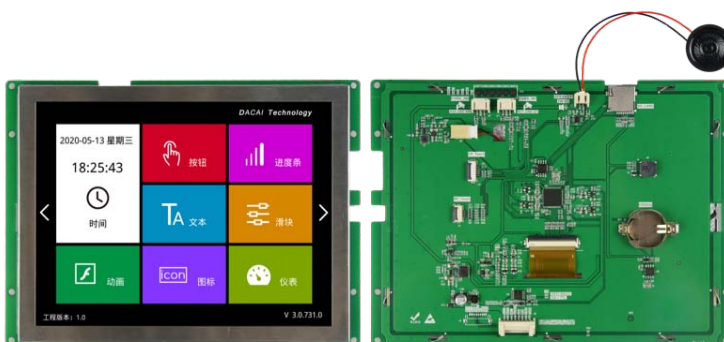
图 1-3 8.0 寸无触摸参考图
