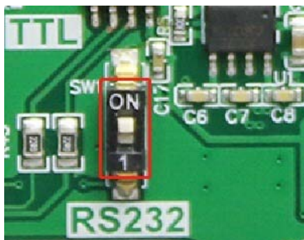
图 8-1 RS232/TTL 电平
