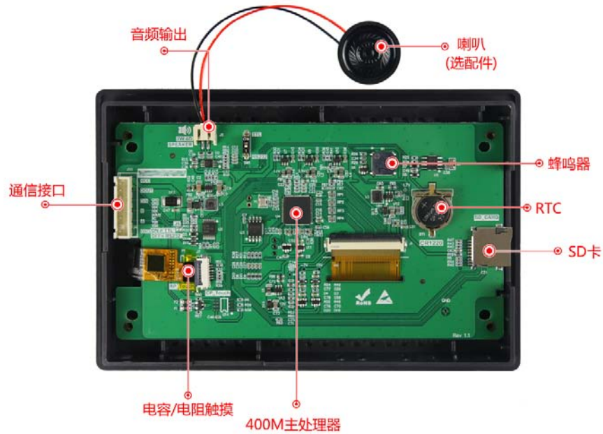
图 1-3 硬件配置图
