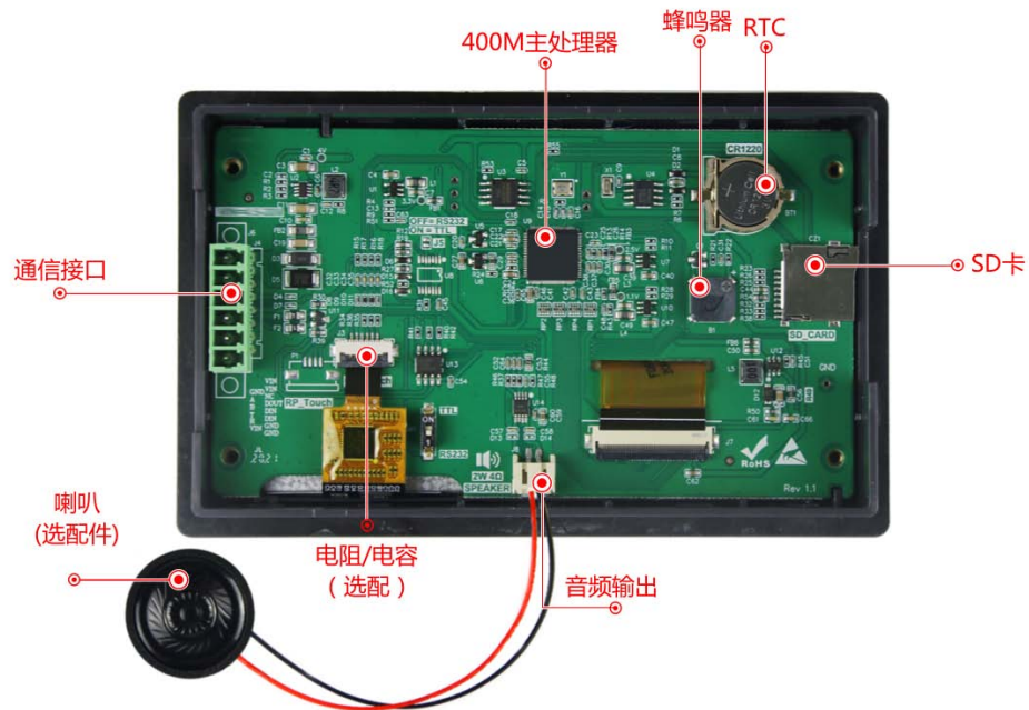
图 1-3 硬件配置图
