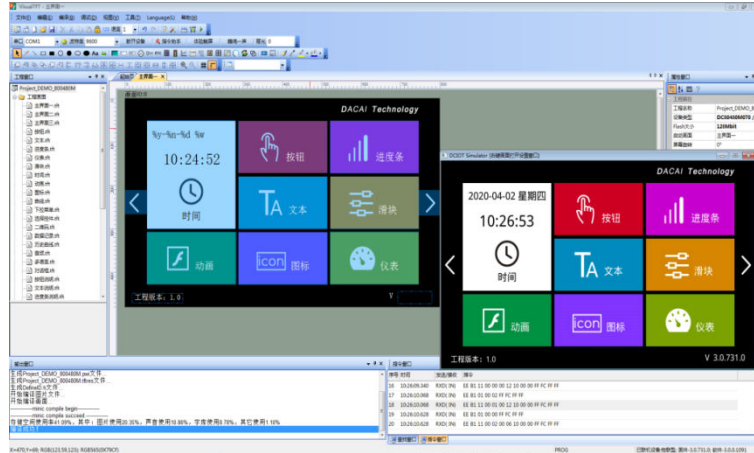
图 12-1 VisualTFT 主界面
