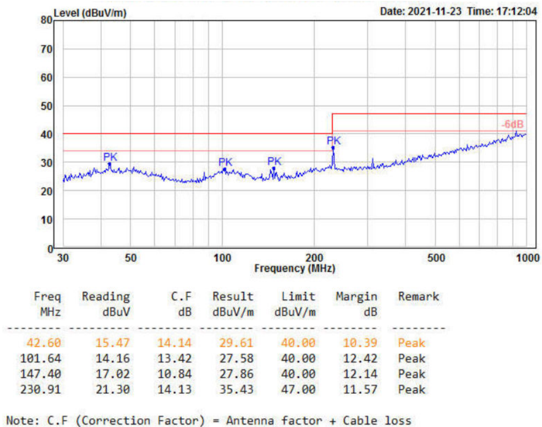
图 6-6 辐射测试水平方向
