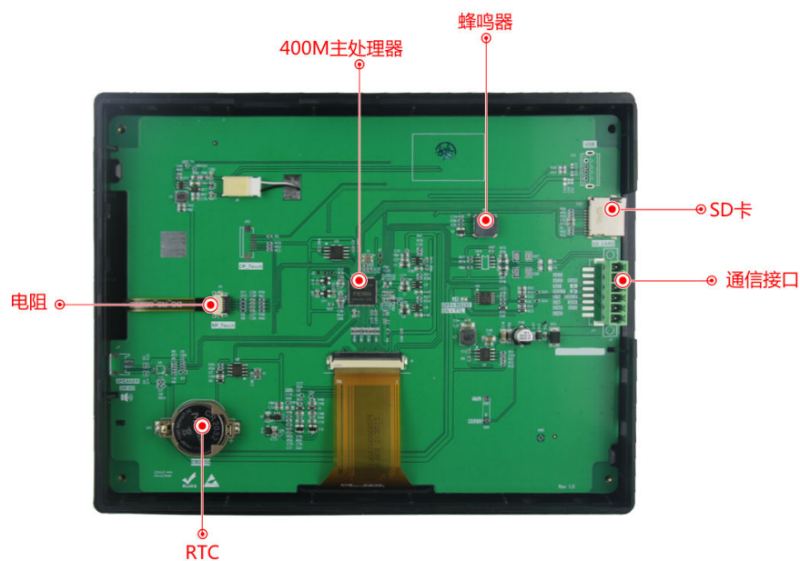
图 1-2 硬件配置图
