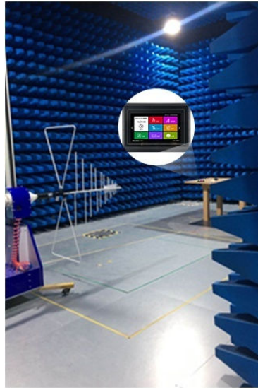
图 6-5 辐射测试图
