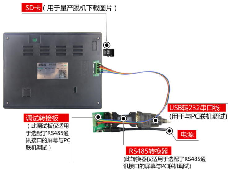
图 1-4 RS485 调试工具图
