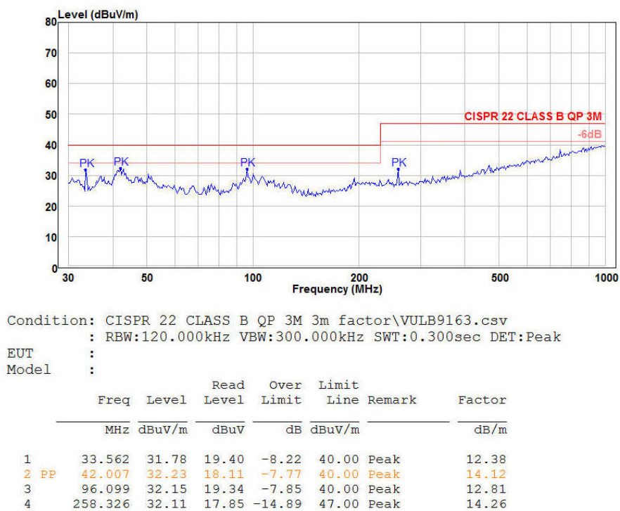
图 3-7 辐射测试垂直方向
