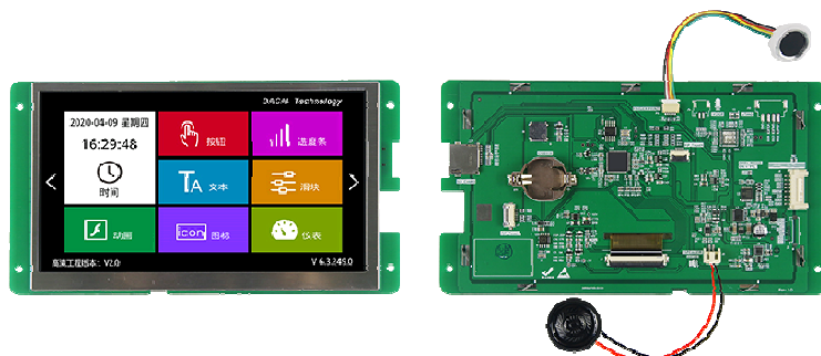
图 1-3 7.0 寸无触摸参考图
