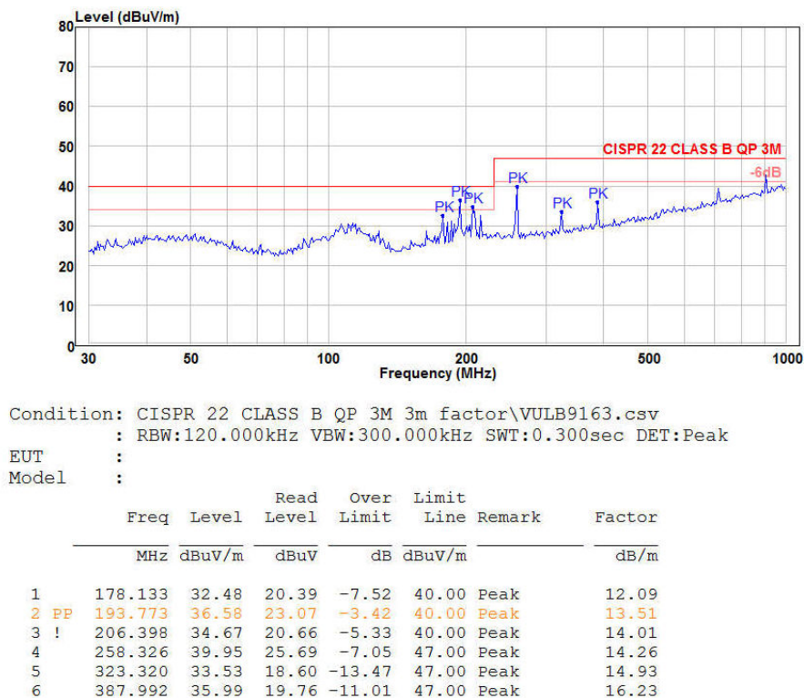
图 3-6 辐射测试水平方向
