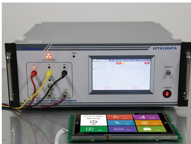
图 3-4 群脉冲测试图
