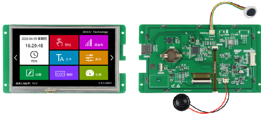
图 1-1 7.0 寸电阻触摸参考图
