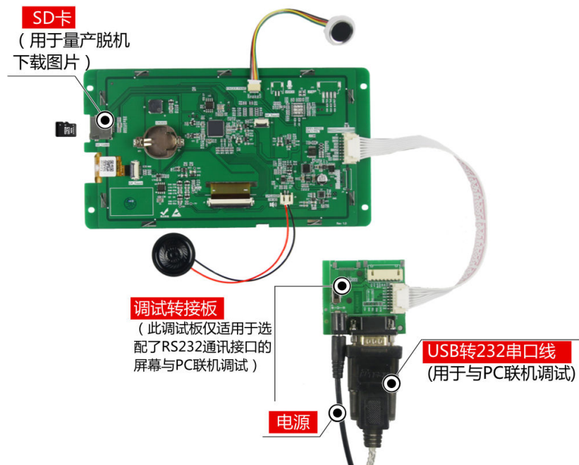
图 1-5 调试工具图
