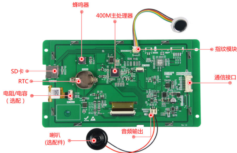
图 1-4 硬件配置图
