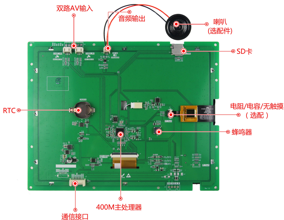
图 1-4 硬件配置图
