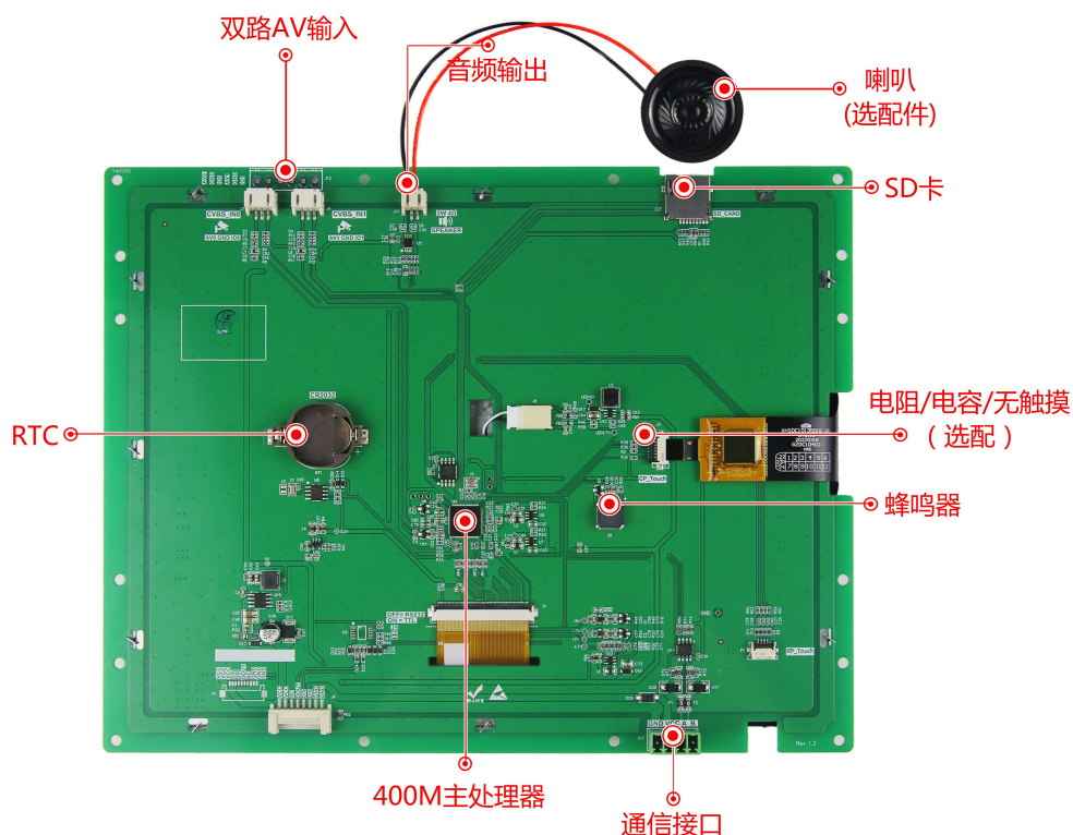
图 1-4 硬件配置图
