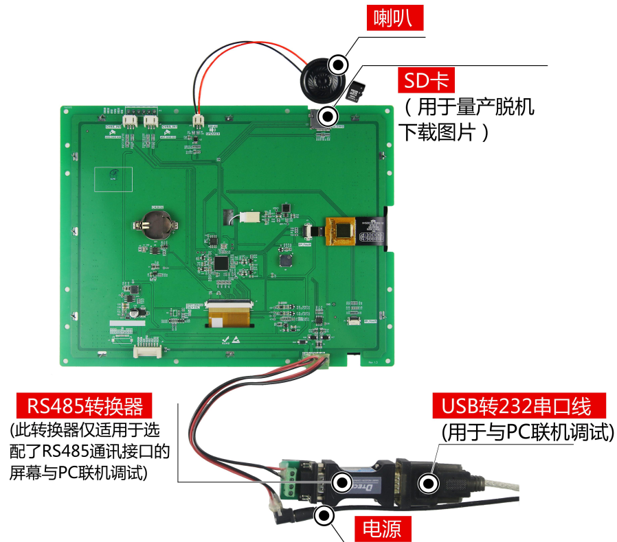
图 1-5 调试工具图
