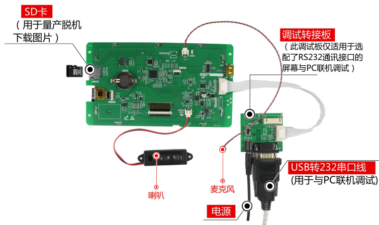
图 1-5 调试工具图
