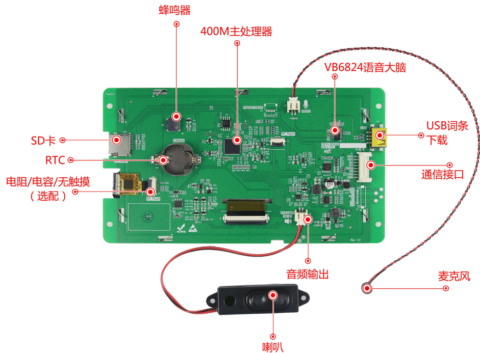
图 1-4 硬件配置图
