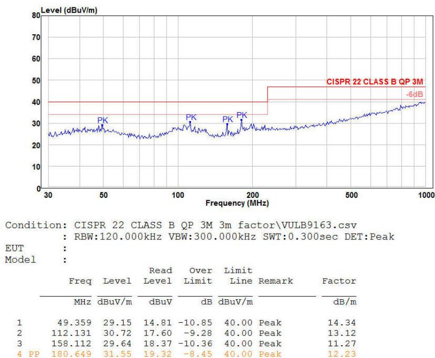
图 3-6 辐射测试水平方向
