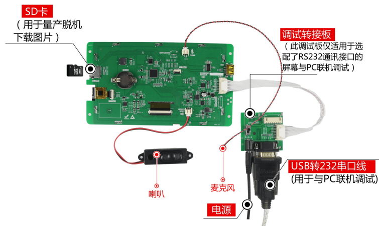
图 1-5 调试工具图
