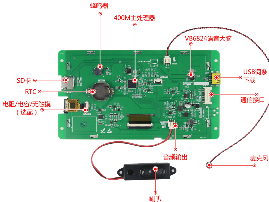
图 1-4 硬件配置图
