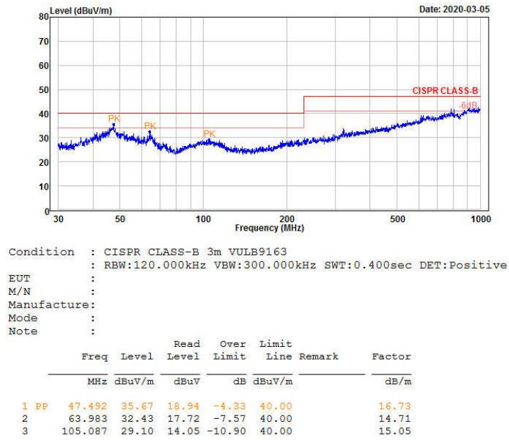
图 5-7 辐射测试垂直方向
