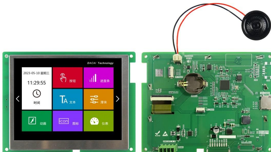
图 1-3 5.6 寸无触摸参考图
