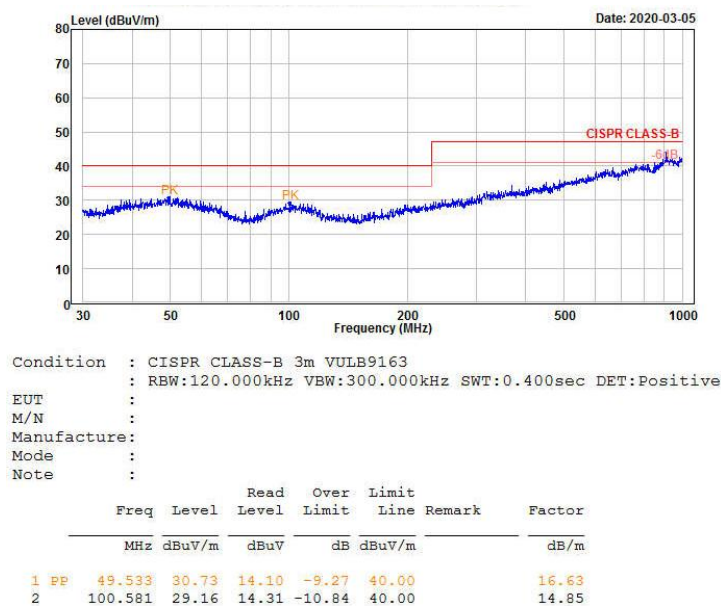
图 5-6 辐射测试水平方向
