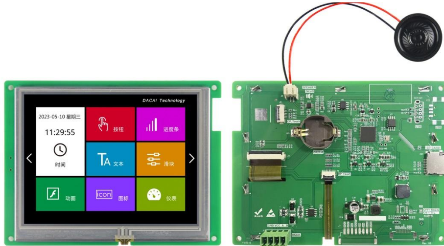
图 1-1 5.6 寸电阻触摸参考图
