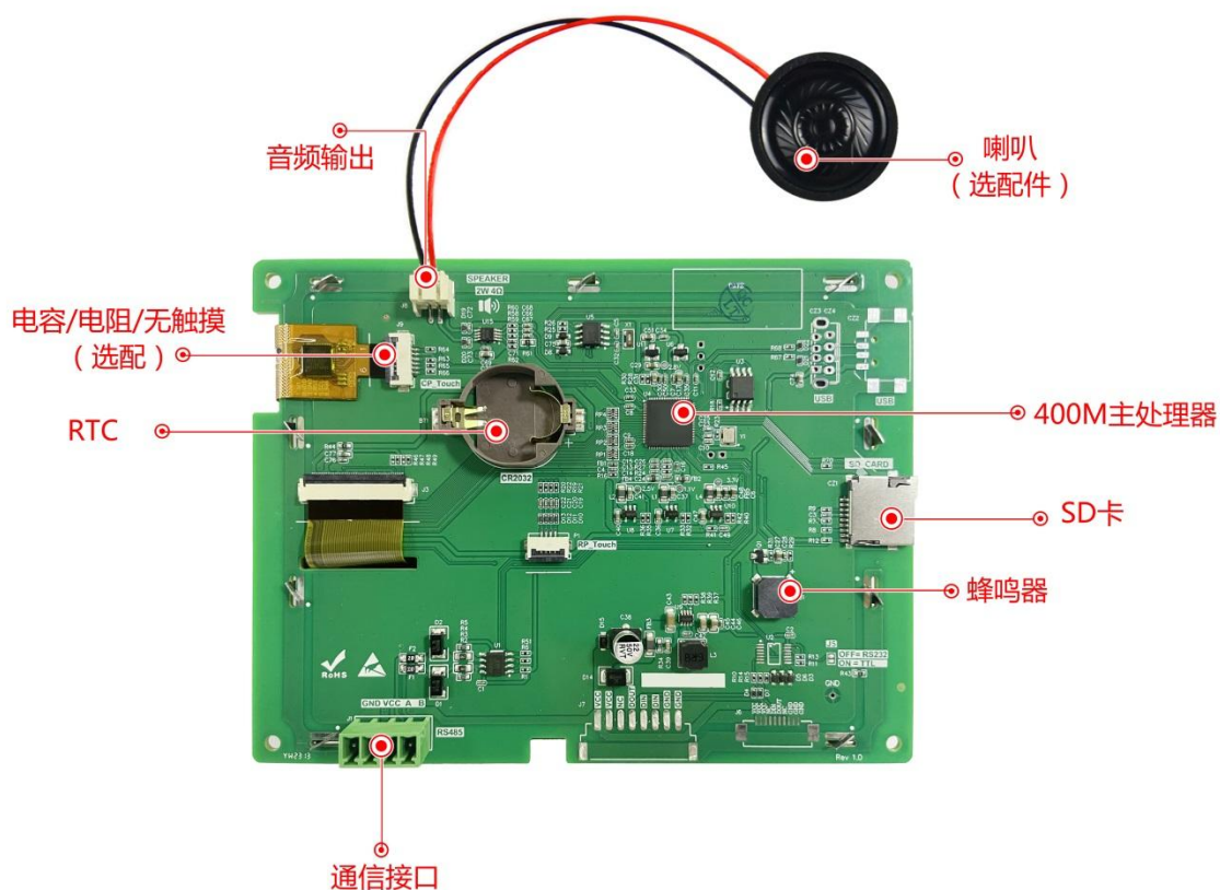
图 1-4 硬件配置图
