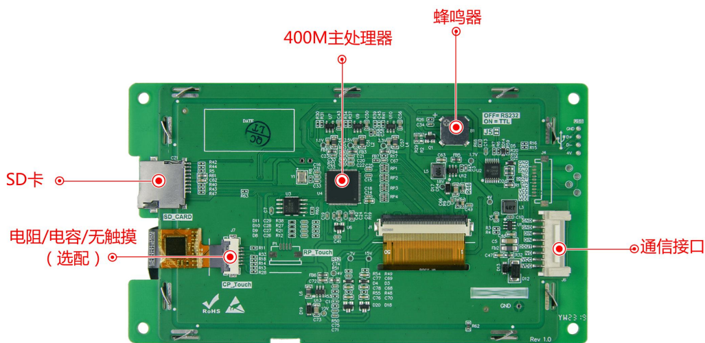
图 1-5 调试工具图
