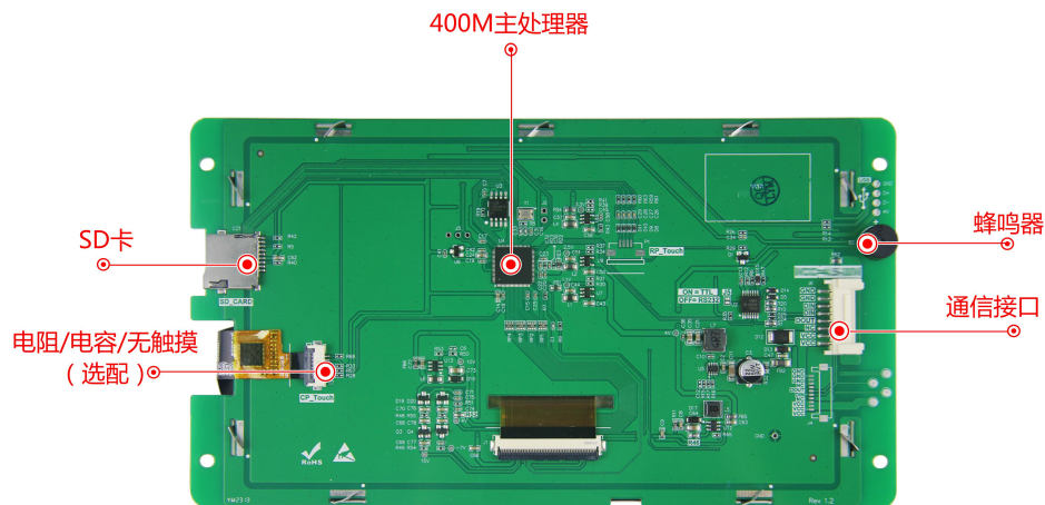
图 1-4 硬件配置图
