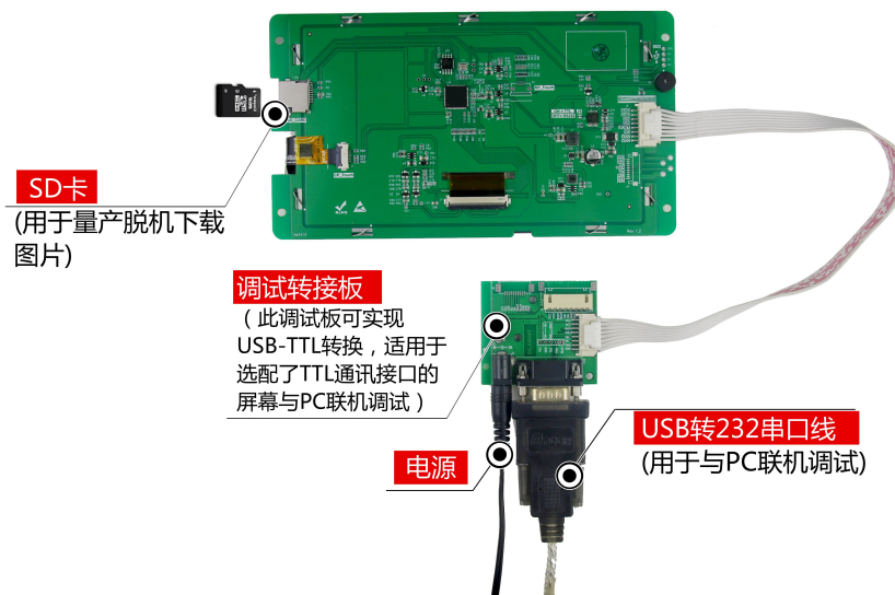
图 1-5 调试工具图
