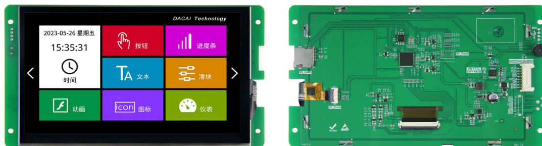
图 1-2 7.0 寸电容触摸参考图
