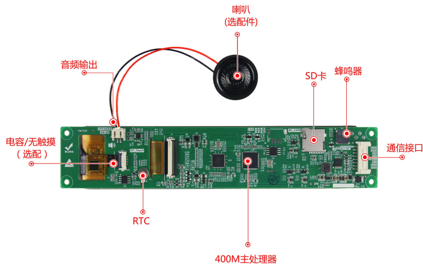
图 1-2 硬件配置图
