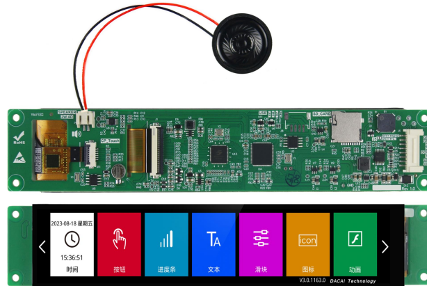
图 1-1 7 寸产品参考图
