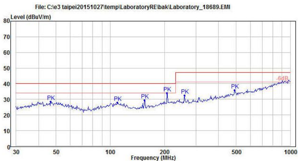
图 5-6 辐射测试水平方向
