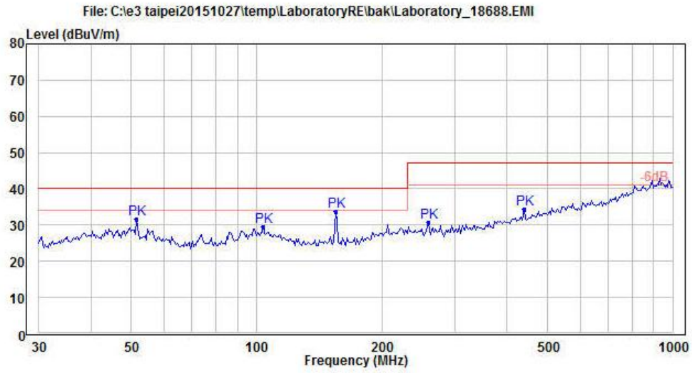
图 5-7 辐射测试垂直方向
