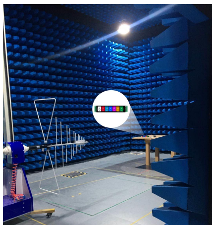
图 5-5 辐射测试图
