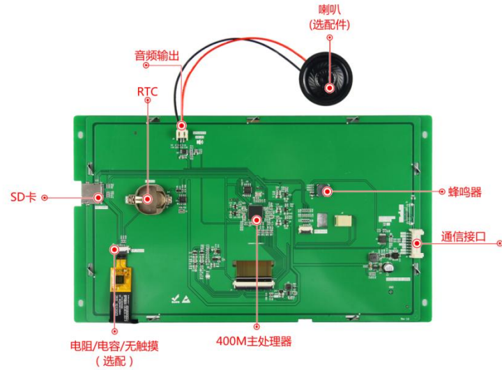
图 1-4 硬件配置图
