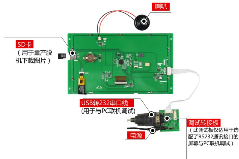
图 1-5 调试工具图
