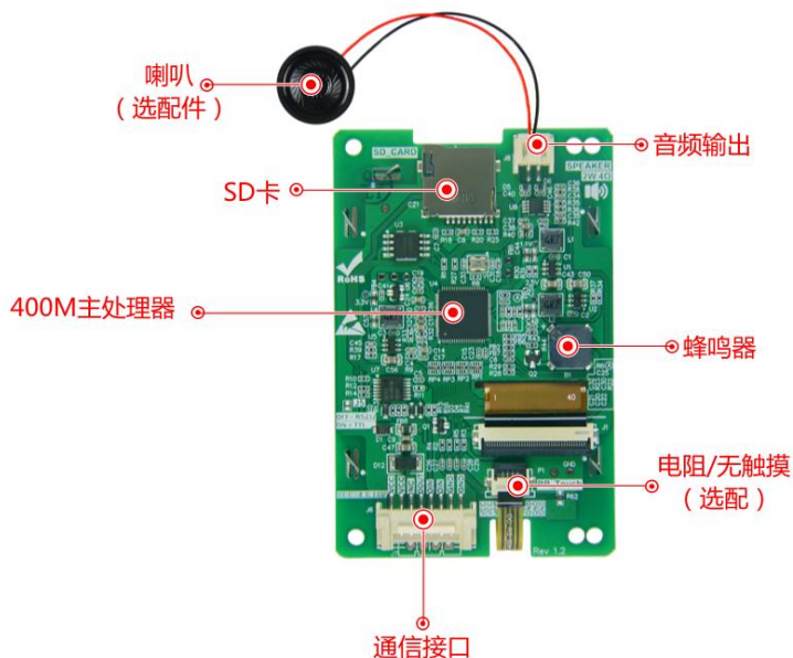
图 1-3 硬件配置图
