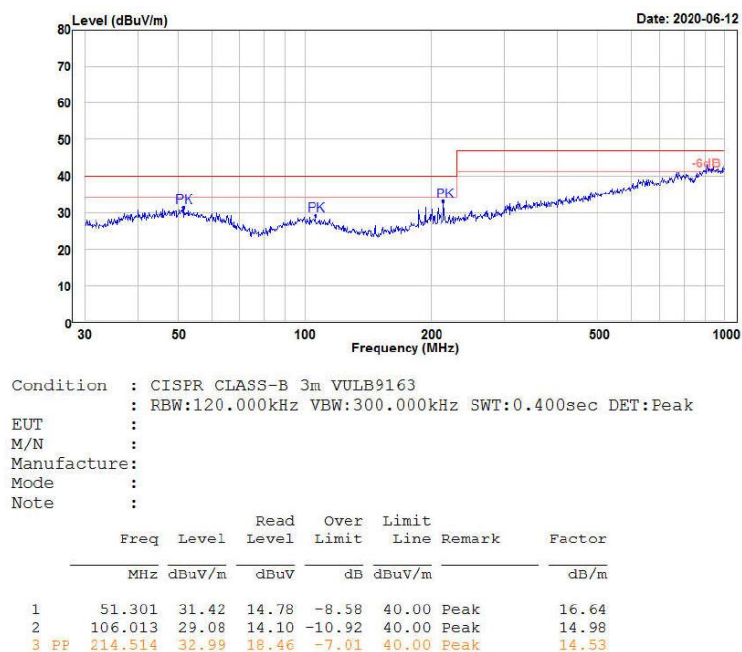
图 5-6 辐射测试水平方向
