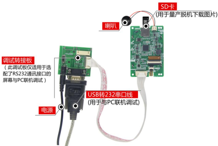
图 1-4 调试工具图
