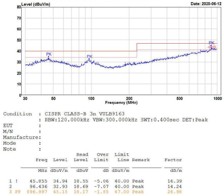
图 5-7 辐射测试垂直方向
